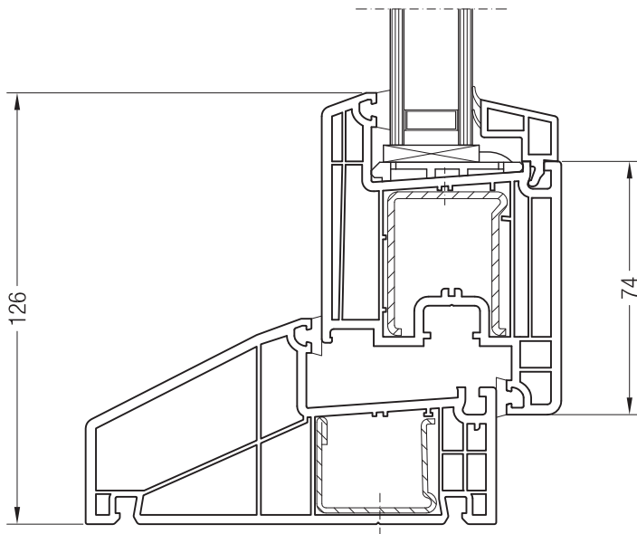
Коробка 60/120, 1550001 и створка Z 74, 1550510
