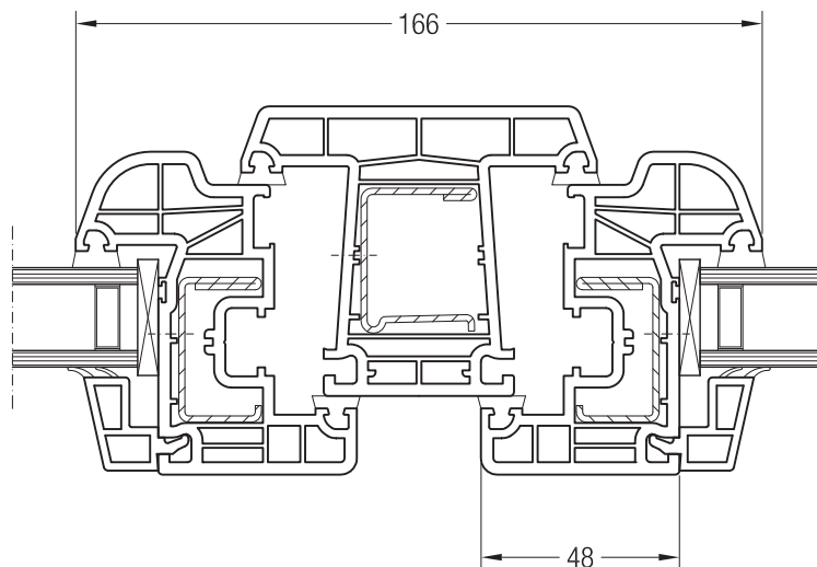
Импост 86, 1550020 и створка 48 круглая, 1550481
