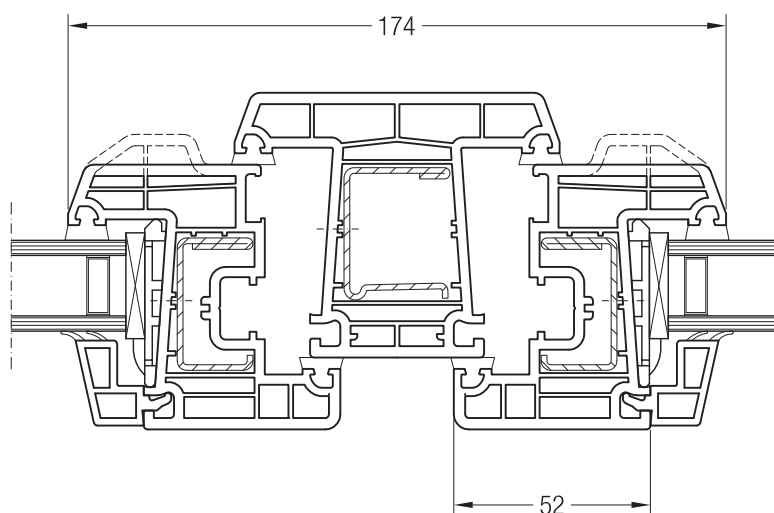
Импост 86, 1550020 и створка Z 52, 1550480 или створка A 52, 1550040
