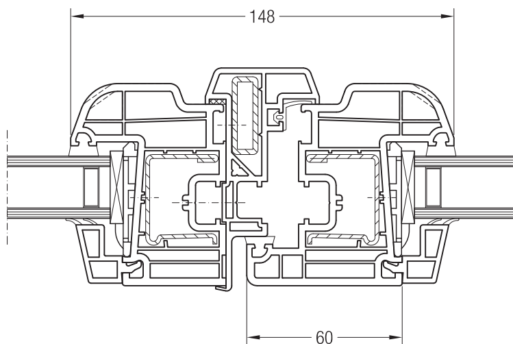
Штульп 70, 1550085 и створка A 60, 1550050 или створка 60 круглая, 1550060
