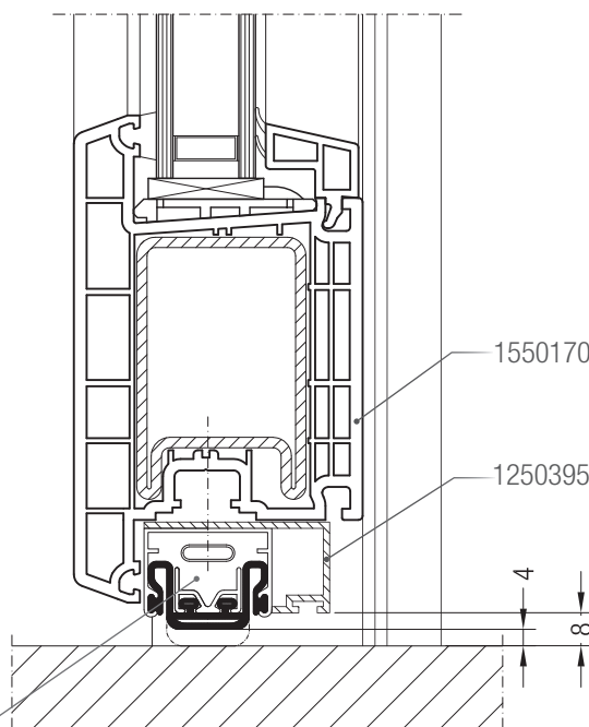
Входная дверь с открыванием наружу
