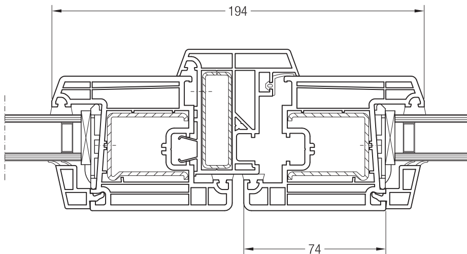
Ложный импост 70, 1550775 и створка Z 74, 1550510
