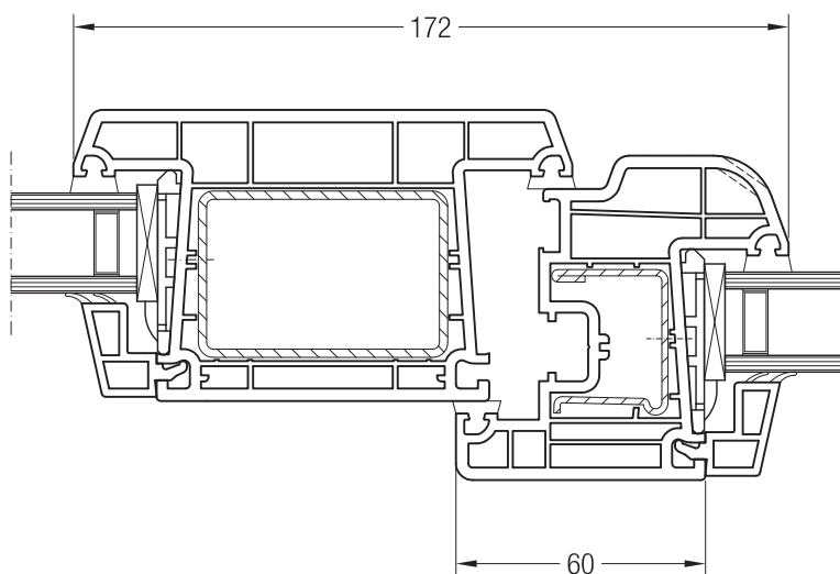
Импост 120, 1550780 и створка A 60, 1550050 или створка 60 круглая, 1550060
