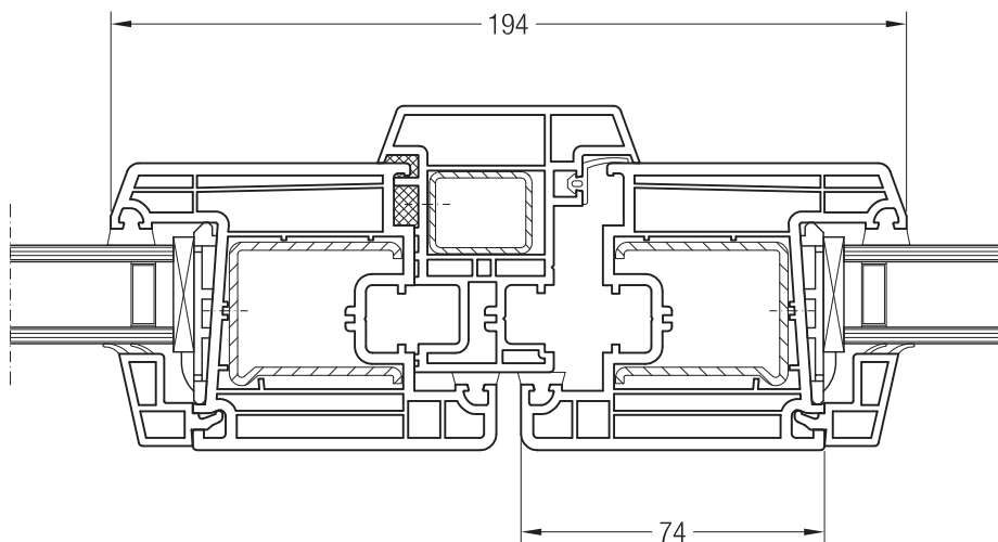
Ложный импост №1, 1550535 и створка Z 74, 1550510
