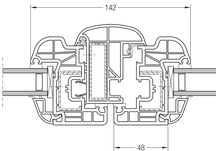
Ложный импост 70 круглый, 1550536 и створка 48 круглая, 1550481
