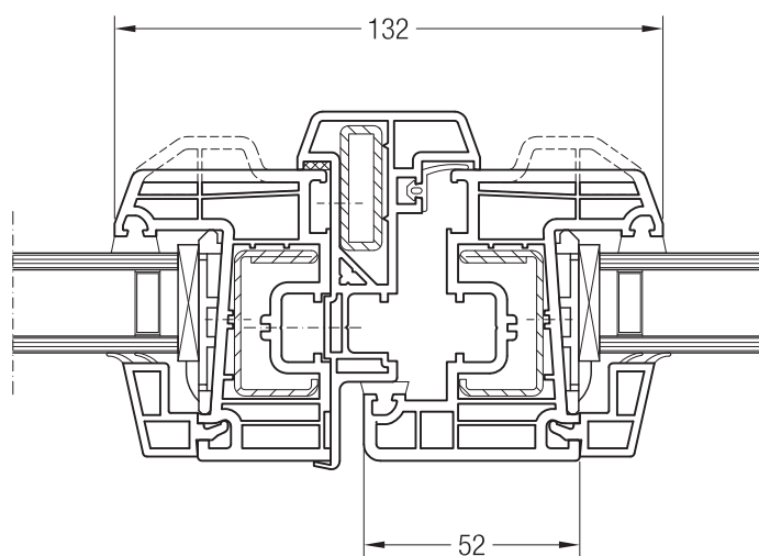
Штульп 70, 1550085 и створка Z 52, 1550480 или створка A 52, 1550040
