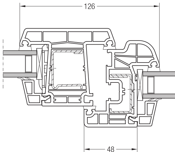
Импост 86, 1550020 и створка 48 круглая, 1550481
