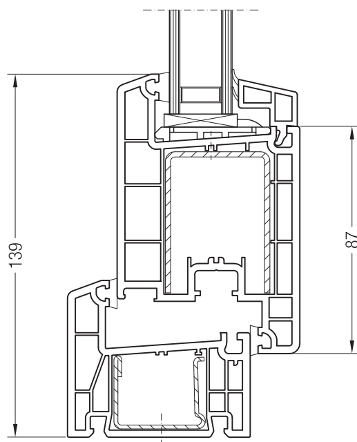
Коробка 60 DK, 1550101 и створка Z 87, 1550760
