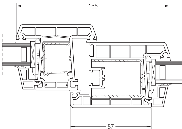
Импост 86, 1550020 и створка Z 87, 1550760
