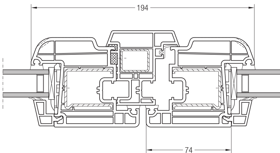
Ложный импост №1, 1550535 и створка A 74, 1550390 или створка 74 круглая, 1550070
