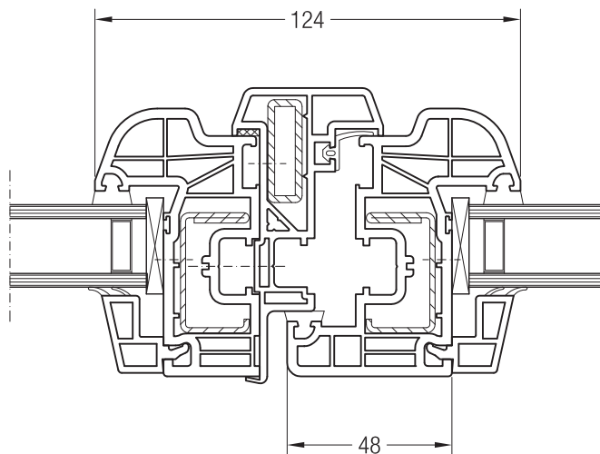
Штульп 70, 1550085 и створка 48 круглая, 1550481
