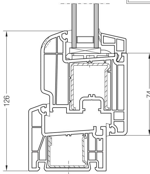
Коробка 60 DK, 1550101 и створка A 74, 1550390 или створка 74 круглая, 1550070
