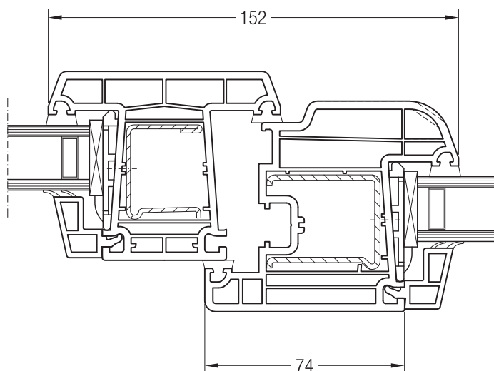
Импост 86, 1550020 и створка A 74, 1550390 или створка 74 круглая, 1550070
