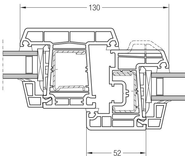
Импост 86, 1550020 и створка Z 52, 1550480 или створка A 52, 1550040
