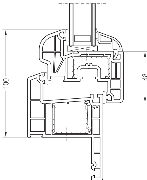
Коробка 60/40, 1550790 и створка 48 круглая, 1550481
