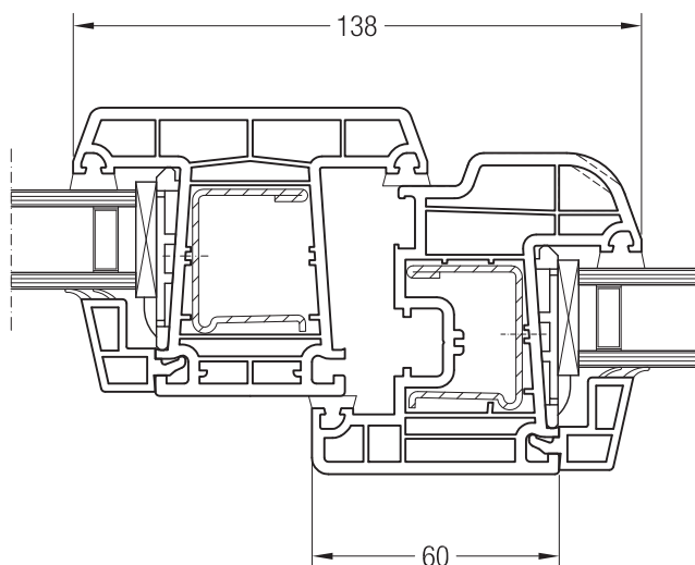
Импост 86, 1550020 и створка A 60, 1550050 или створка 60 круглая, 1550060
