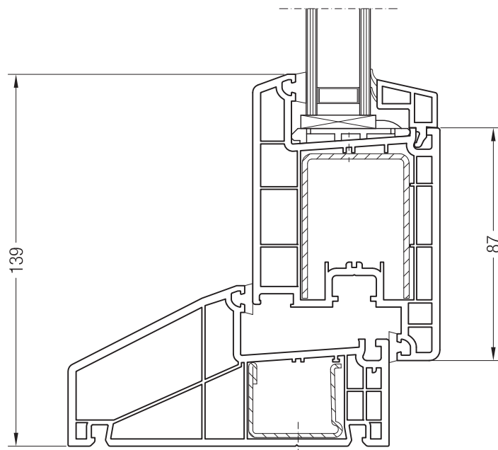
Коробка 60/120, 1550001 и створка Z 87, 1550760
