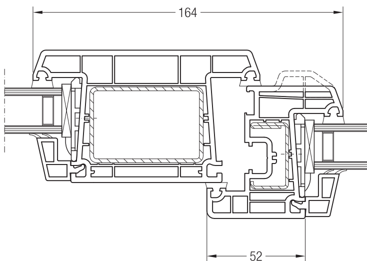
Импост 120, 1550780 и створка Z 52, 1550480 или створка A 52, 1550040
