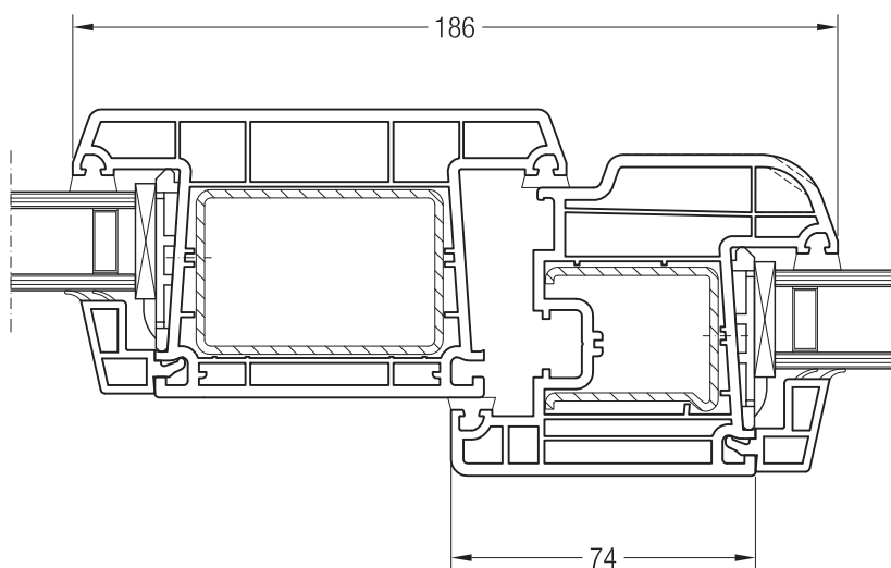
Импост 120, 1550780 и створка A 74, 1550390 или створка 74 круглая, 1550070
