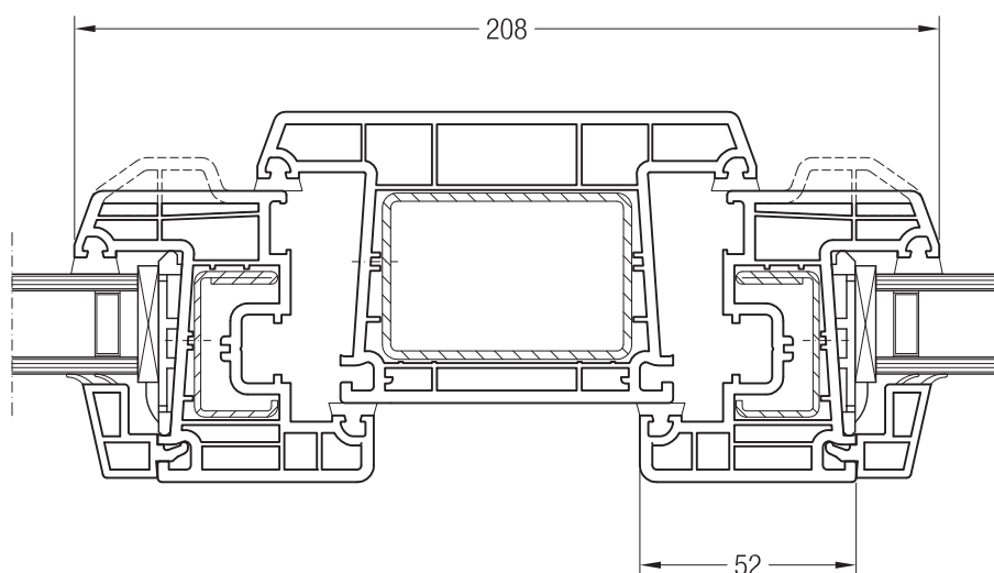
Импост 120, 1550780 и створка Z 52, 1550480 или створка A 52, 1550040
