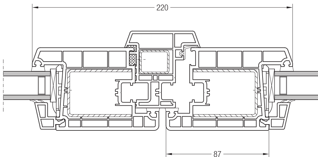
Ложный импост №1, 1550535 и створка Z 87, 1550760
