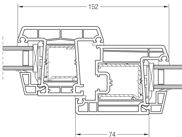
Импост 86, 1550020 и створка Z 74, 1550510
