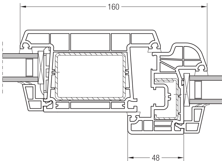
Импост 120, 1550780 и створка 48 круглая, 1550481
