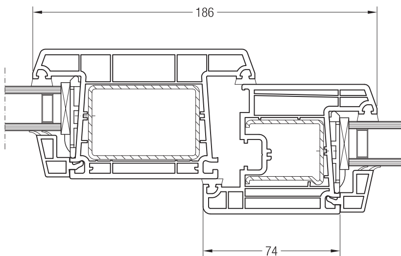
Импост 120, 1550780 и створка Z 74, 1550510
