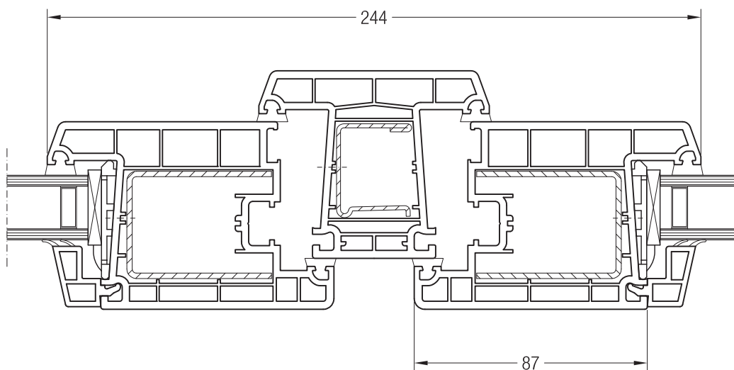
Импост 86, 1550020 и створка Z 87, 1550760
