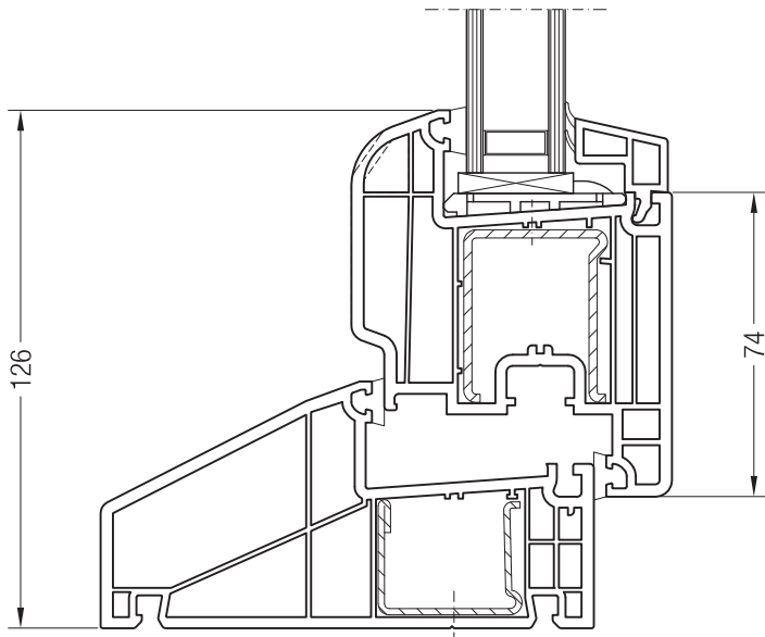
Коробка 60/120, 1550001 и створка A 74, 1550390 или створка 74 круглая, 1550070
