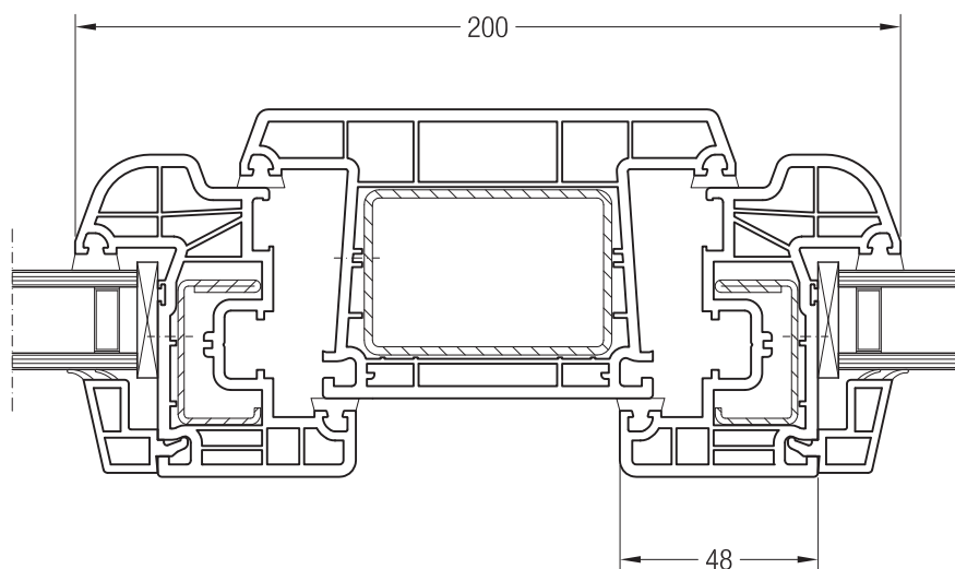
Импост 120, 1550780 и створка 48 круглая, 1550481
